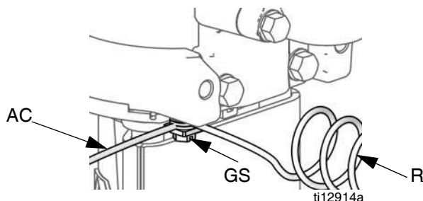
FIG. 3. Vis et fil de terre
