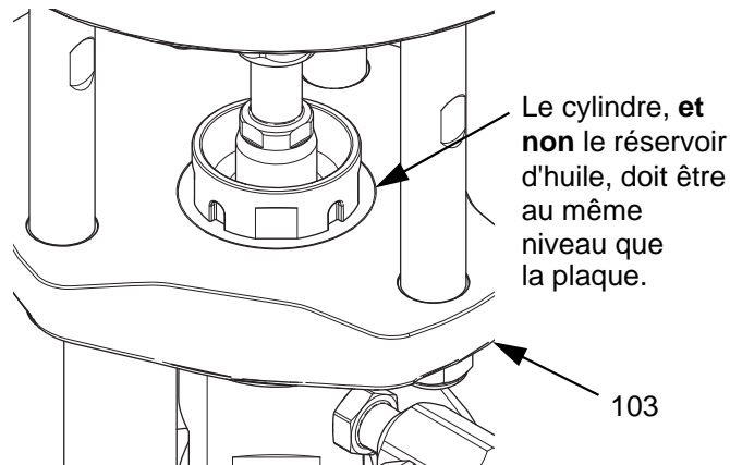
FIG. 6 : Alignez le cylindre et la plaque d'adaptateur.
