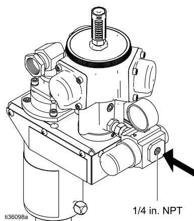
Figure 2 Connexion d'air d'alimentation
