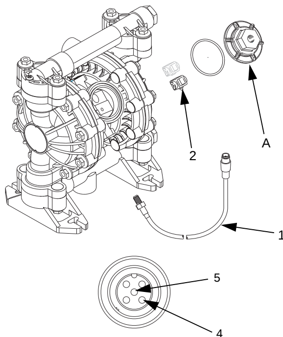
Connecteur de câbles Broches 1-3 inutilisées
