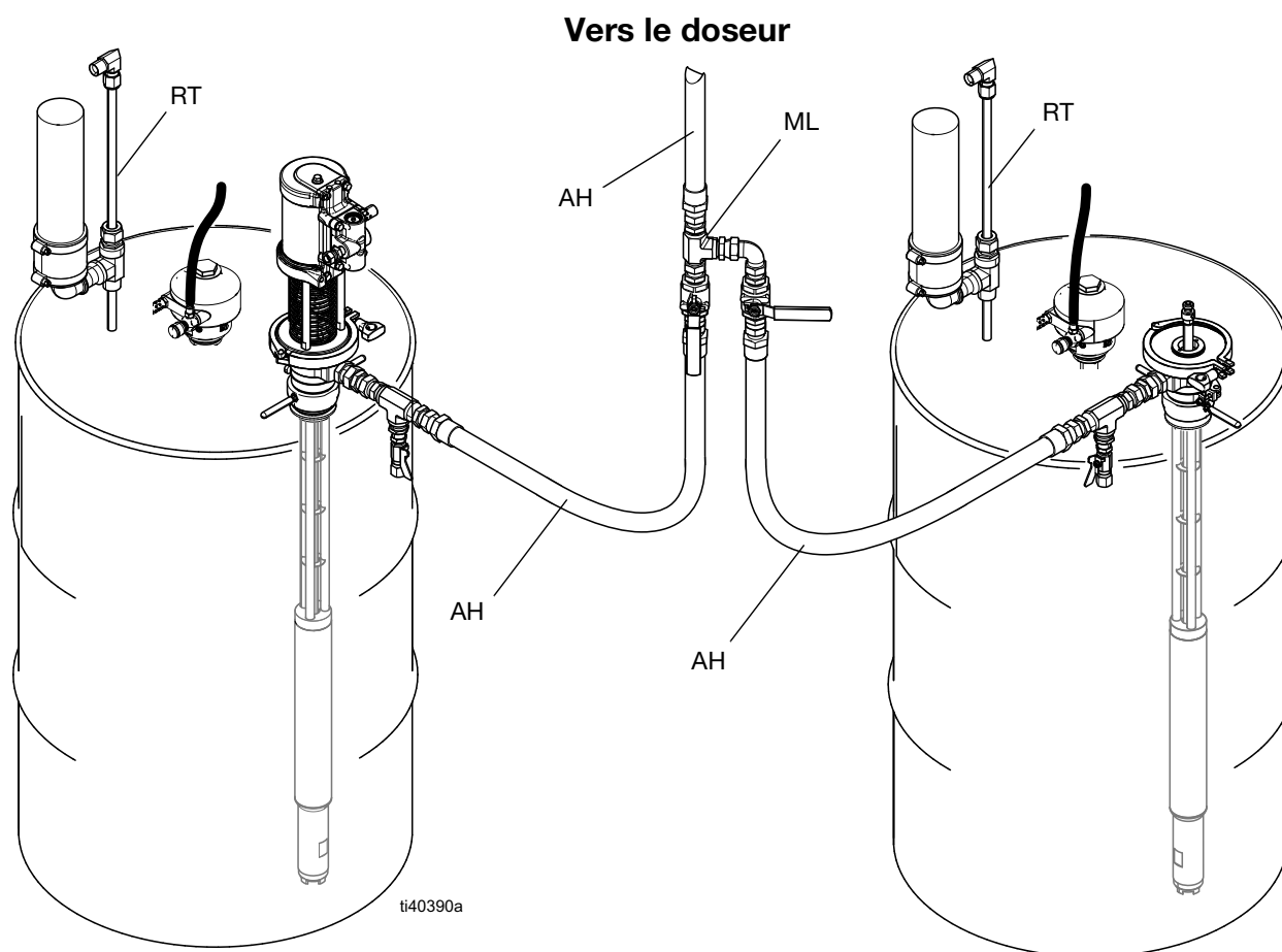
FIG. 4: Installation type de bas de pompe multiples
