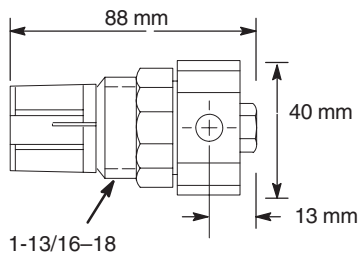
Modèle 110318, C06117 (orifice de 1/4")
