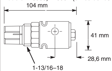
Modèle 171937 (orifice de 1/2")
