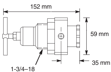
Modèle 110234 (orifice de 3/8")
