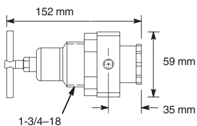
Modèle 104266, 104267 (orifice de 1/2") 113406 (orifice de 1/4")
