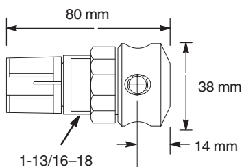
Modèle 110234 (orifice de 3/8")
