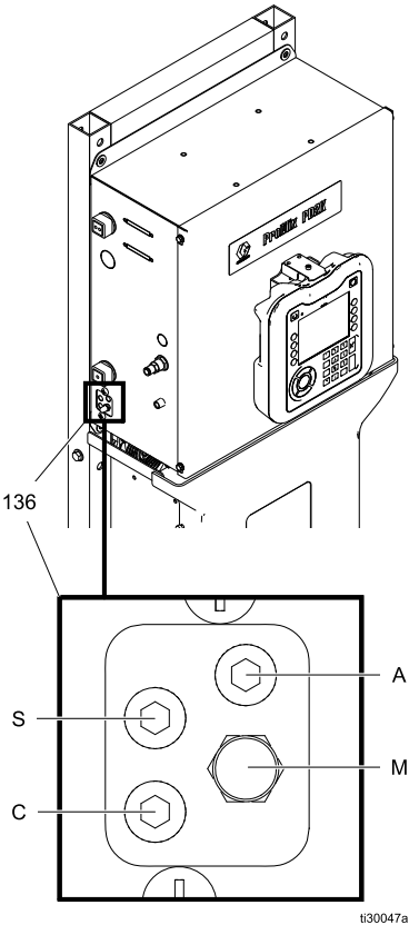
Figure 17 Raccords de l'air d'atomisation et du collecteur d'air Légende
