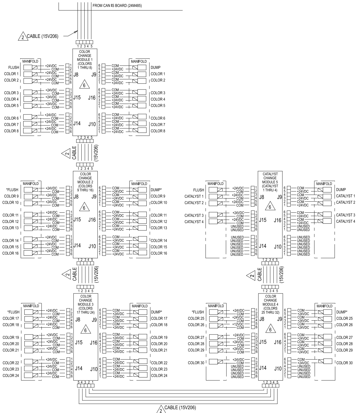
Figure 28 Schéma électrique, feuille 3
