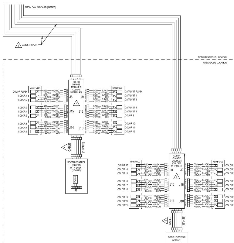
Figure 35 Schéma électrique, feuille 3, partie 2
