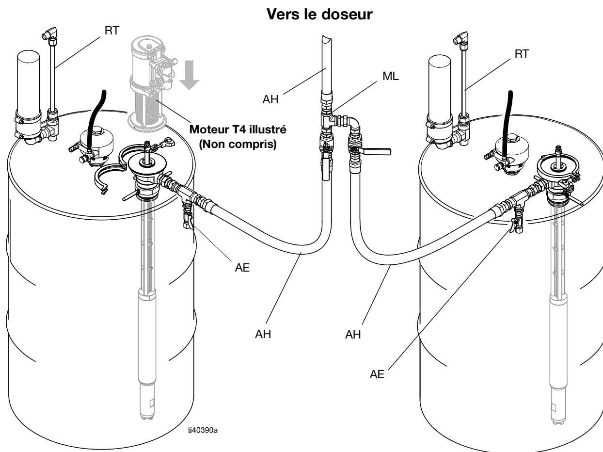
FIG. 1: Installation type de bas de pompe multiples
