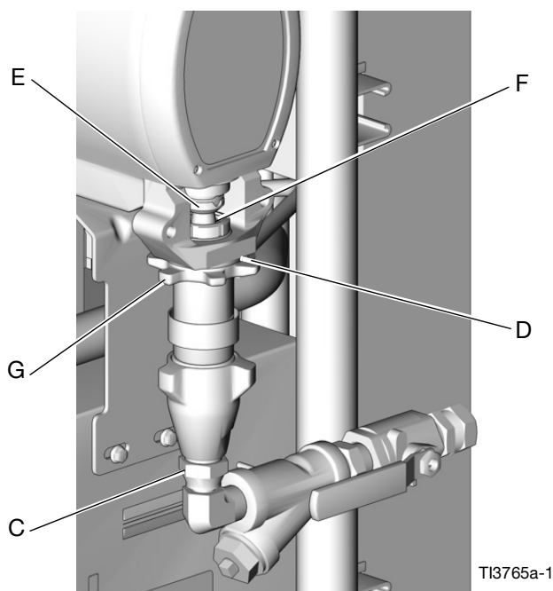
FIG. 2 Débranchement de la pompe B
