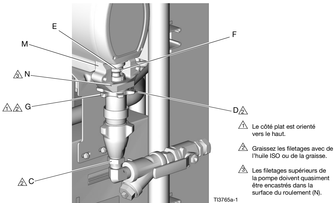
FIG. 3 Rebrancher la pompe B
