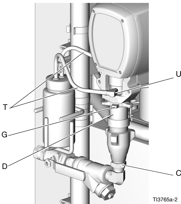
FIG. 1 Débranchement de la pompe A
