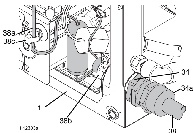
FIG. 9 : Cordon/câble d'alimentation (moteurs F-2 et F-4)
