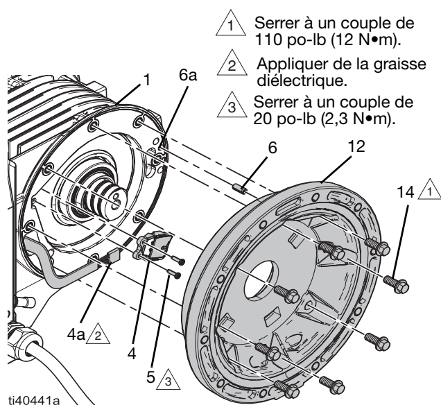
FIG. 17 : Capteur du moteur
