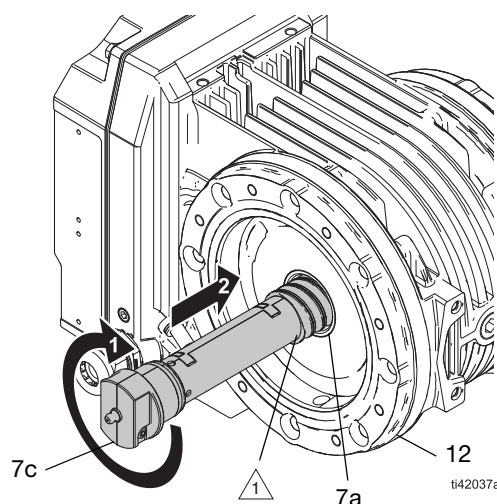
Fig. 22 : Insertion de l'outil de graissage du rotor
