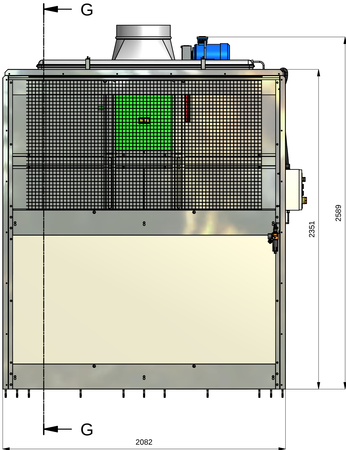
Vista frontale
