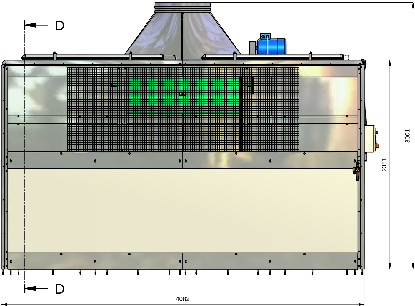
Vista anteriore
