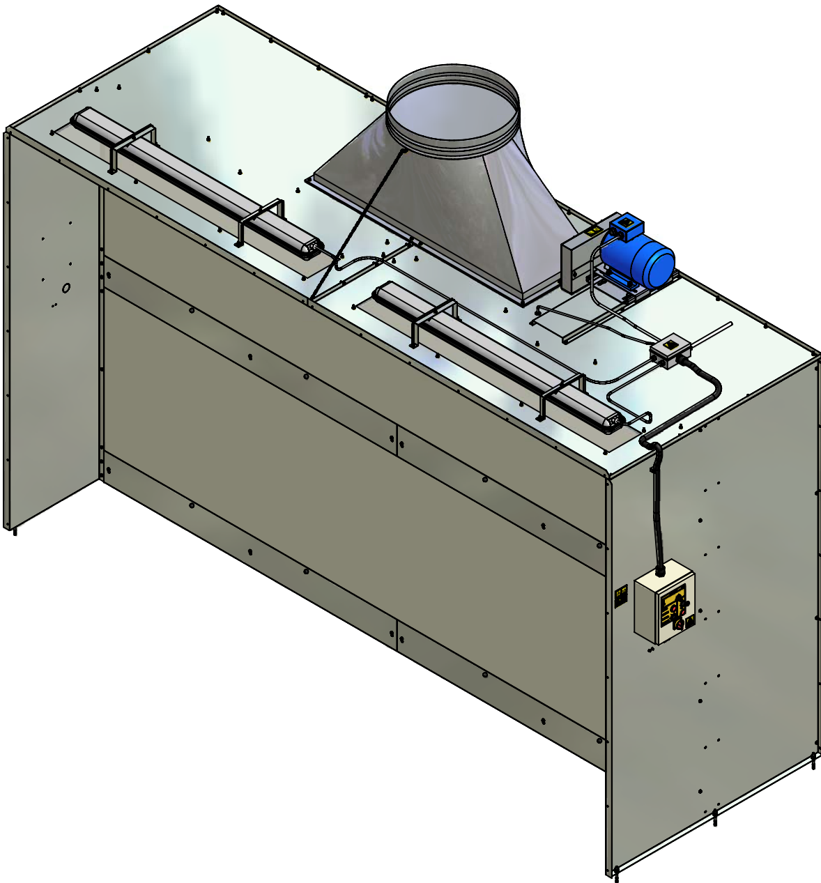
Vista prospettica
