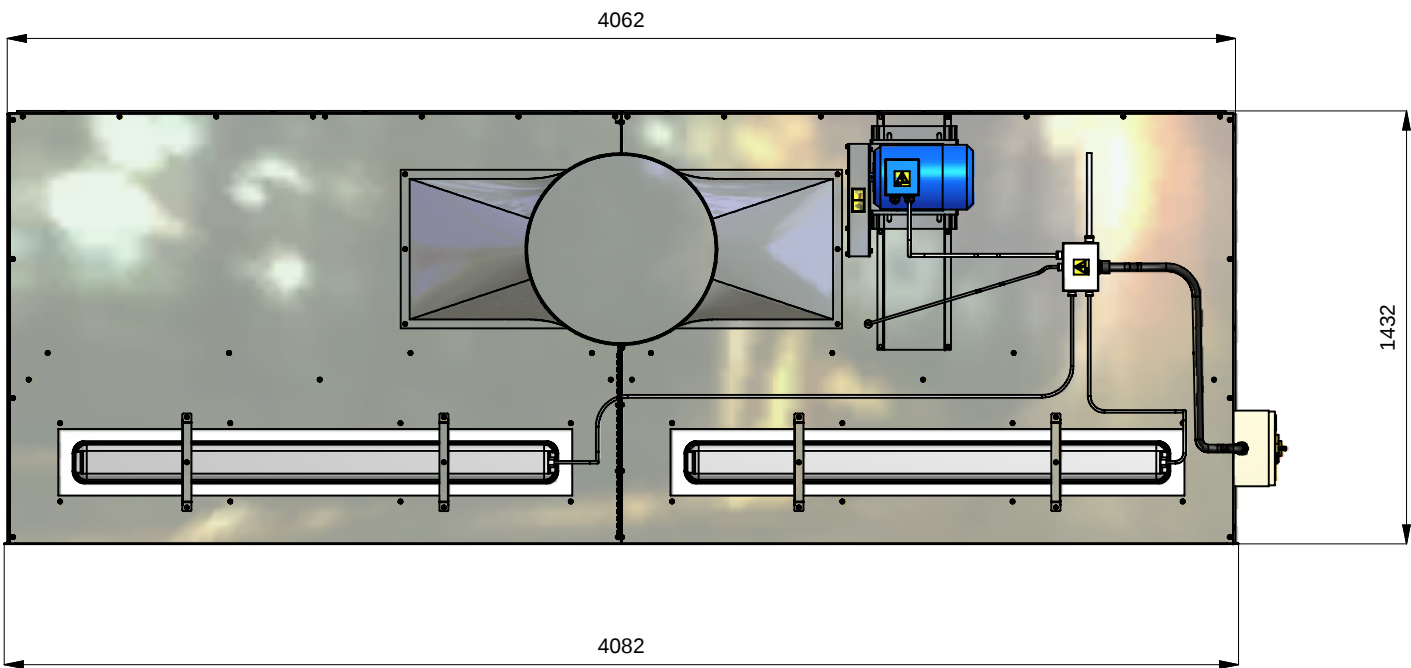
Vista dall'alto
