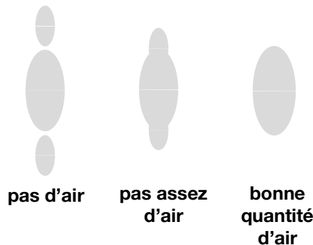
FIG. 6. Problèmes de jet de pulvérisation
