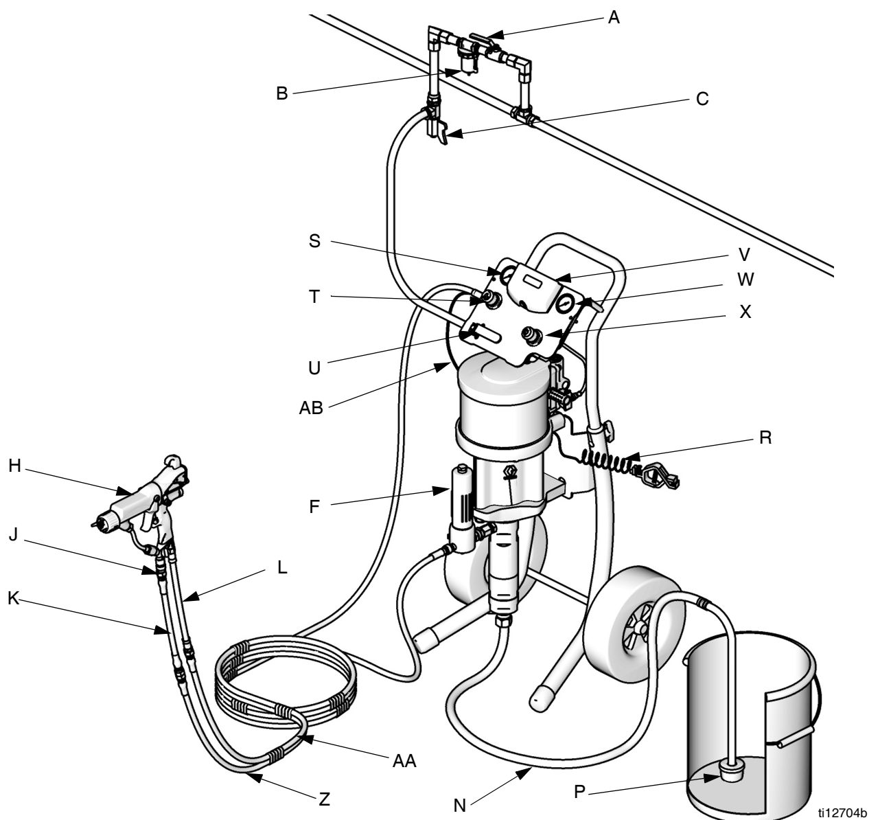
FIG. 1. Installation type, modèle G30C76 à température ambiante illustré.
