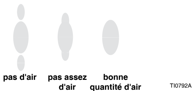
FIG. 8. Problèmes de jet de pulvérisation
