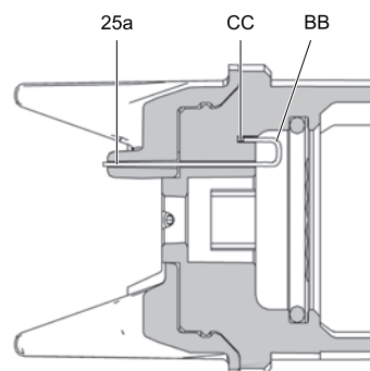
Figure 24 Remplacement de l'électrode
