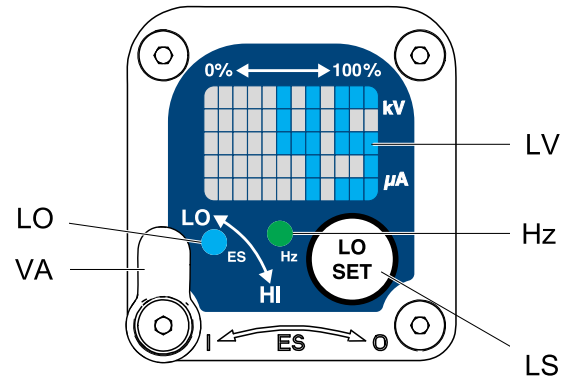
Figure 4 Écran du paramètre de basse tension (déverrouillé)
