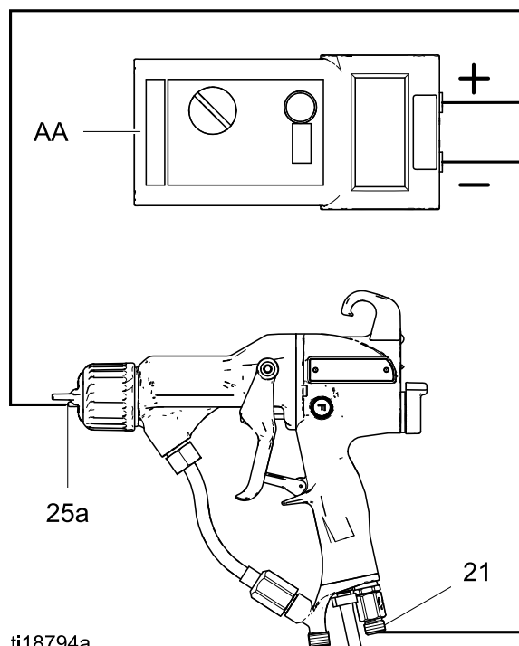
Figure 17 Test de résistance du pistolet
