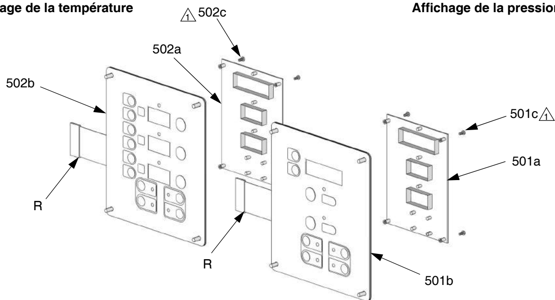
FIG. 13. Module d'affichage
