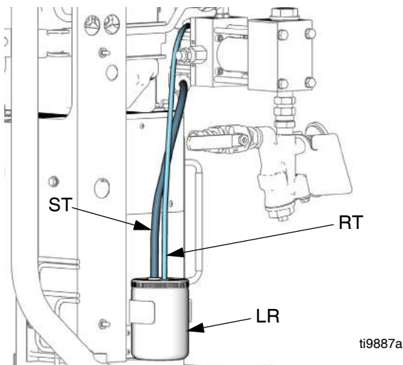
FIG. 15. Système de pompe de graissage
