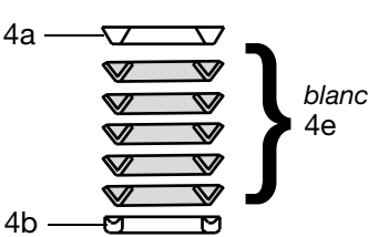
Joint de piston : Lèvres vers le haut
