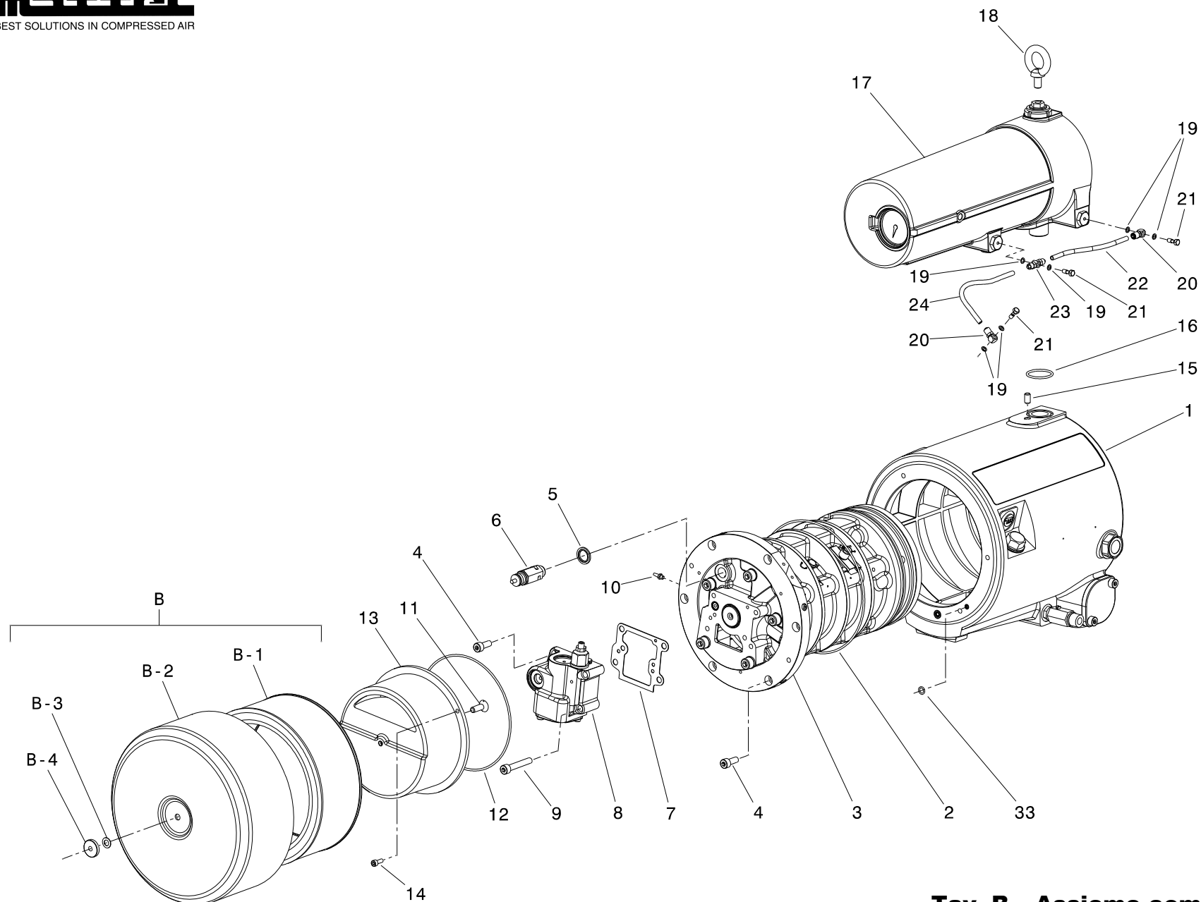
Tav. B – Assieme compressore Compressor assembly
