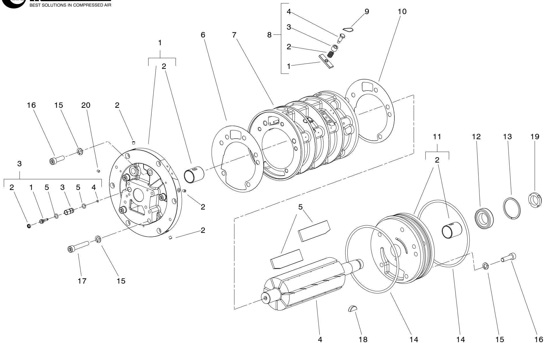
Tav. D – Assieme rotore-statore Rotor-stator assembly
